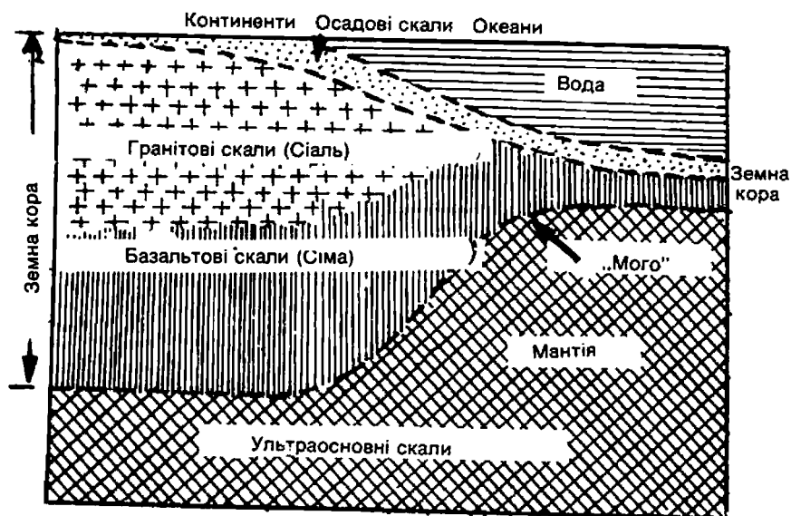
Різниця в глибині земної кори під континентами й океанами.
