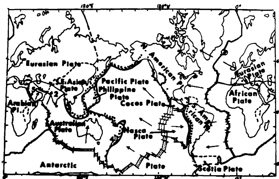
Розміщення поодиноких плит земної кори й напрямки їх пересування та розміщення вулканічних полос на Землі.
