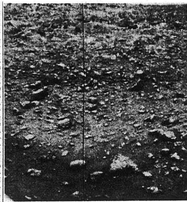
Чорно-біла репродукція першої кольорової фотознімки поверхні Марса.
